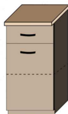
40H шир. 400мм. вис. 850мм. гл. 445/600мм.
