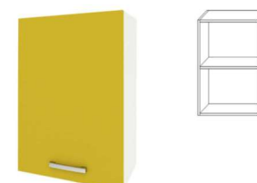
50,40,30B шир. 500,400,300мм. гл. 305мм. вис. 718мм.
