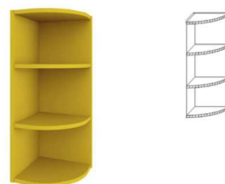
30BK3 шир. 300мм. гл. 305мм. вис. 718мм.
