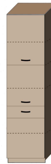
60Н Пенал шир. 600мм. вис. 2133мм. гл. 540мм.
