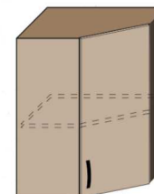
KB 60x60 шир. 550x550мм. вис. 718мм. гл. 305мм.
