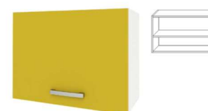
80,60BBC хром шир. 800,600мм. гл. 305мм. вис. 718мм.
