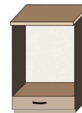
60HДух шир. 600мм. вис. 850мм. гл. 445/600мм.
