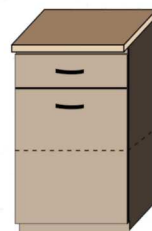
50H шир. 500мм. вис. 850мм. гл. 445/600мм.
