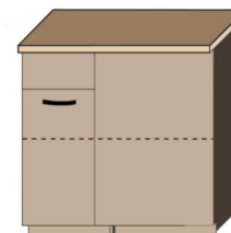
KH 100x60 шир. 950мм. вис. 850мм. гл. 445/600мм.
